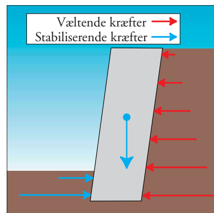
Støttemurens virkemåde. Murens egen vægt og jordtrykket foran muren skal opheve det jordtryk der opstår bag muren.
